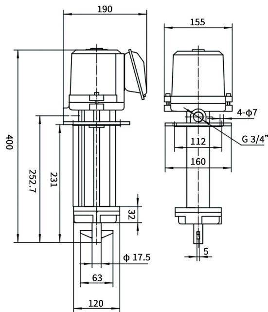
DBJ-200 尺寸图
