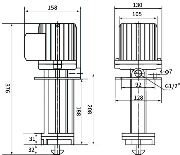
DBJ-90 尺寸图
