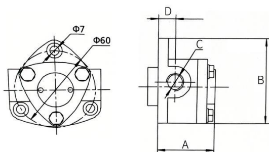
普通泵头尺寸图
