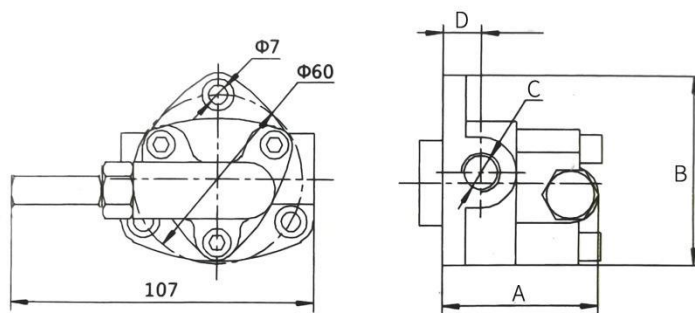
可调式泵头尺寸图
